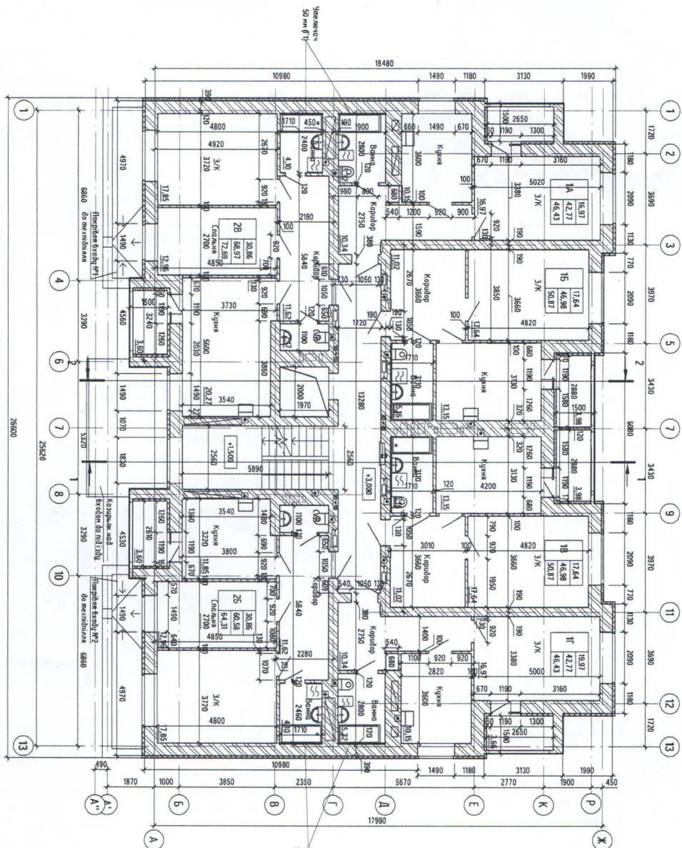
План типового поверху (2-8) М:100
